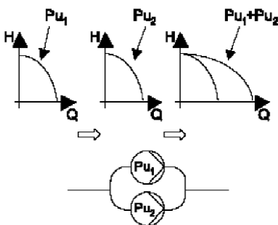
Figura 14. Curvas de capacidad de bombas en paralelo.
