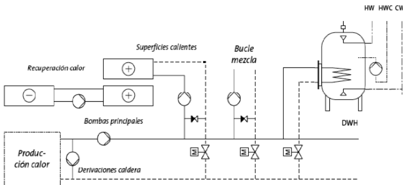
Figura 22. Diferentes tipos de utilizations de bombas de velocidad variable.
