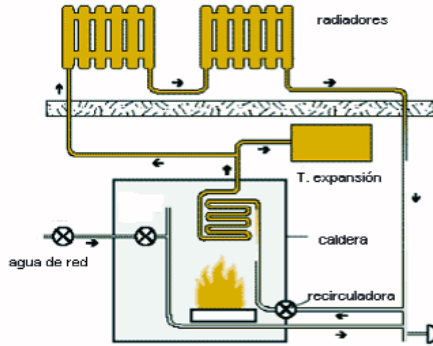
Figura 4. Circuito monotubo.
