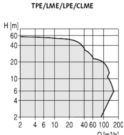
Figura 28. Curva característica con control de velocidad.
