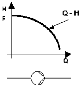
Figura 13. Curva presión-caudal.
