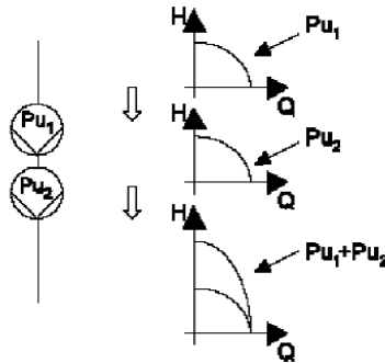
Figura 15. Curvas de capacidad de bombas en serie.
