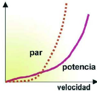
Figura 18. Curvas de Par y Potencia vs velocidad.
