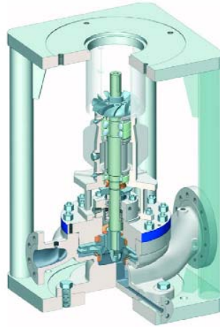
Figura 12. Bomba recirculadora centrífuga.
