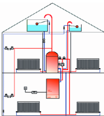
SISTEMA BITUBO RETORNO DIRECTO
