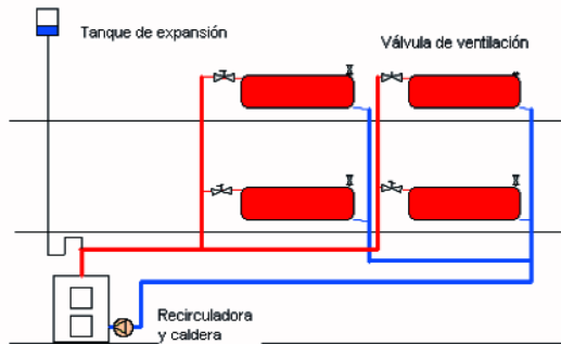
SISTEMA BITUBULAR RETORNO INVERTIDO
