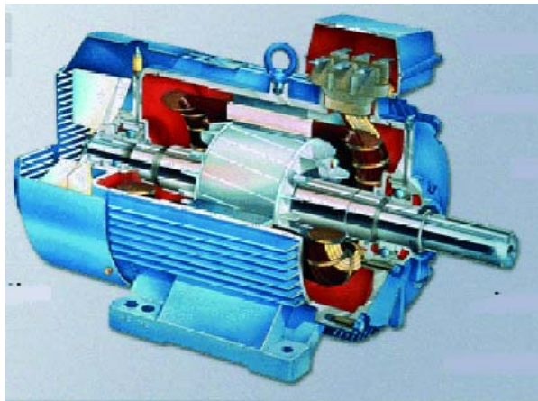
Figura 17. Motor asíncrono.
