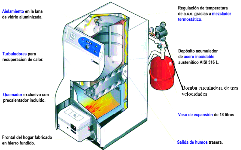
Figura 3. Caldera de gasóleo de pie con bomba de tres velocidades.
